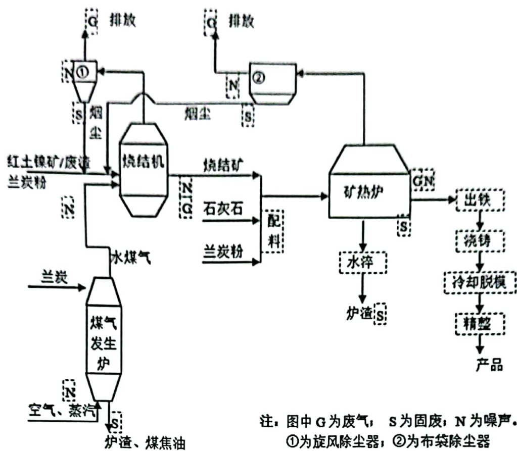
生产工艺流程及产污环节图
