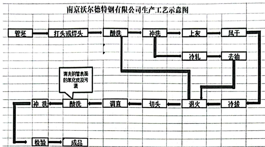
生产工艺流程图：
